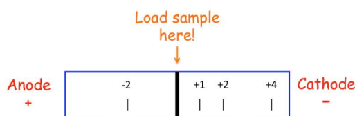
Figure : l'électrophorèse
